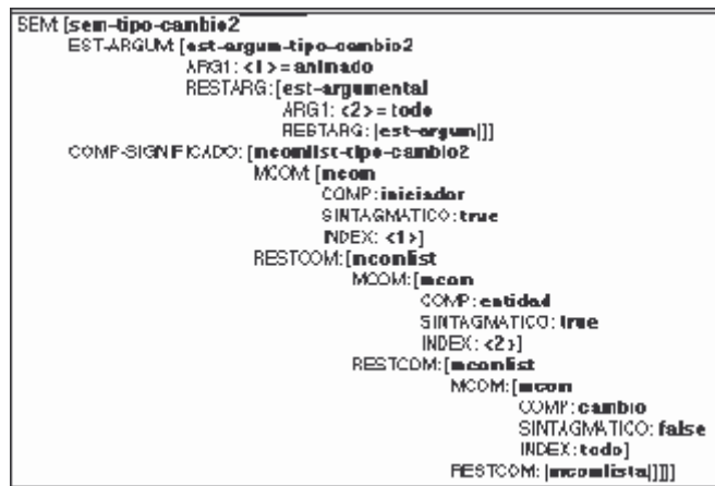
Fig. 2: Semántica de los predicados de cambio del tipo romper
