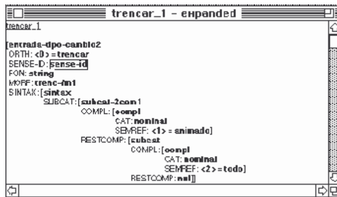
Fig. 3: Componente de subcategorización de los predicados tipo romper
