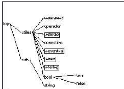
Fig. 1: Jerarquía de tipos
